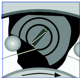
Abb.3 berührungsfreie Position
