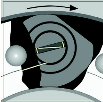
Abb.2 Drehmomentübertragung
