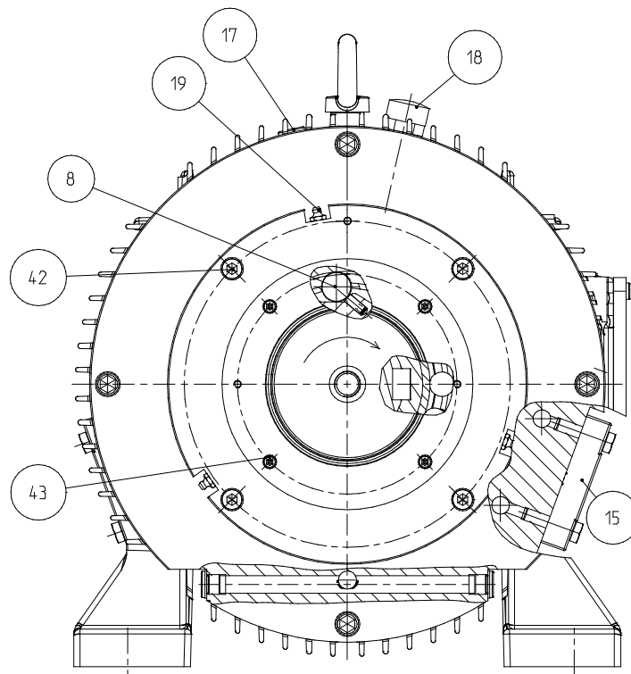
Abb.1a Aufbau
