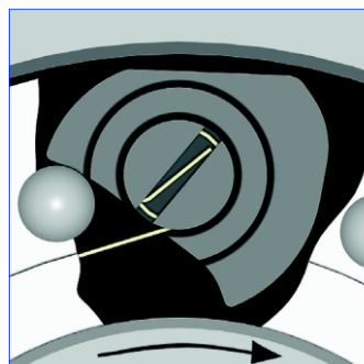
Abb.3 berührungsfreie Position
